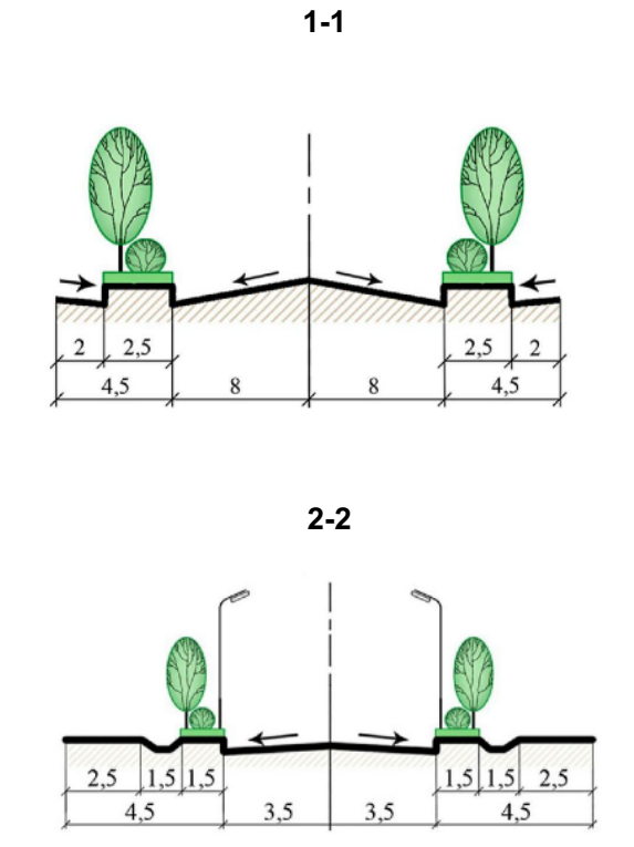
Поперечные профили
